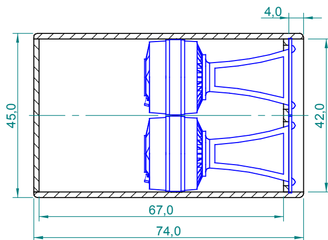
Corte A-A
