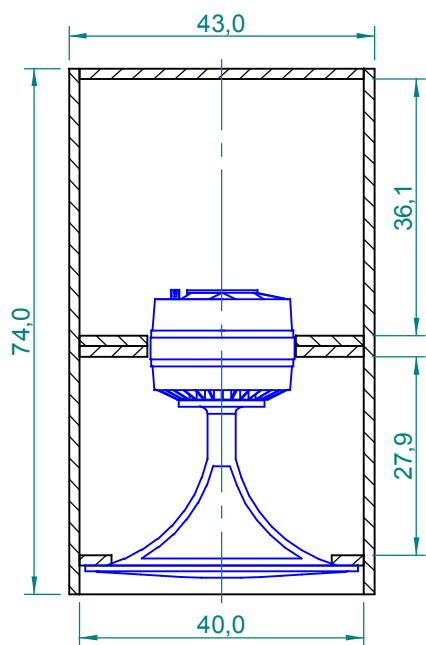
Corte B-B
