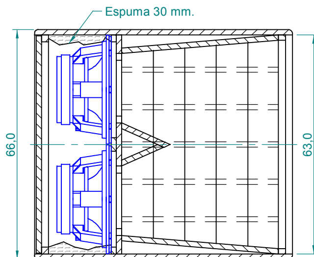
Corte B-B
